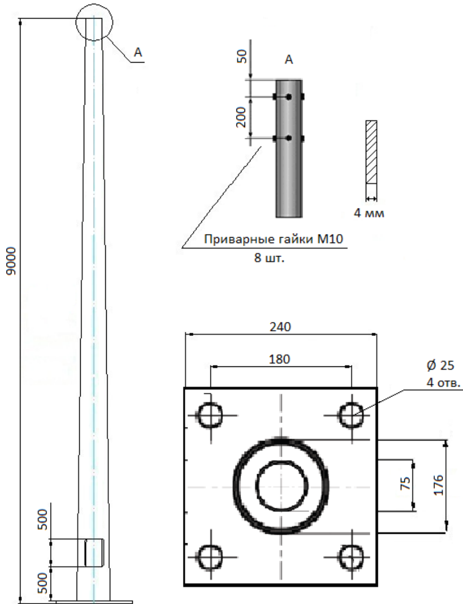
Рис.1 - Габаритные и присоединительные размеры
